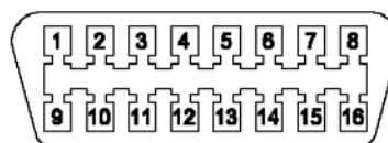
Pinbelegung OBD Buchse, Ansicht von vorne
